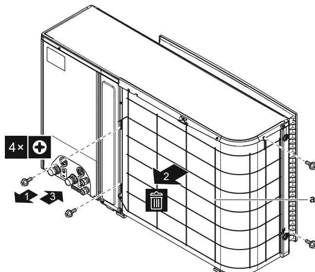
a Iesūkņēšanas restes
