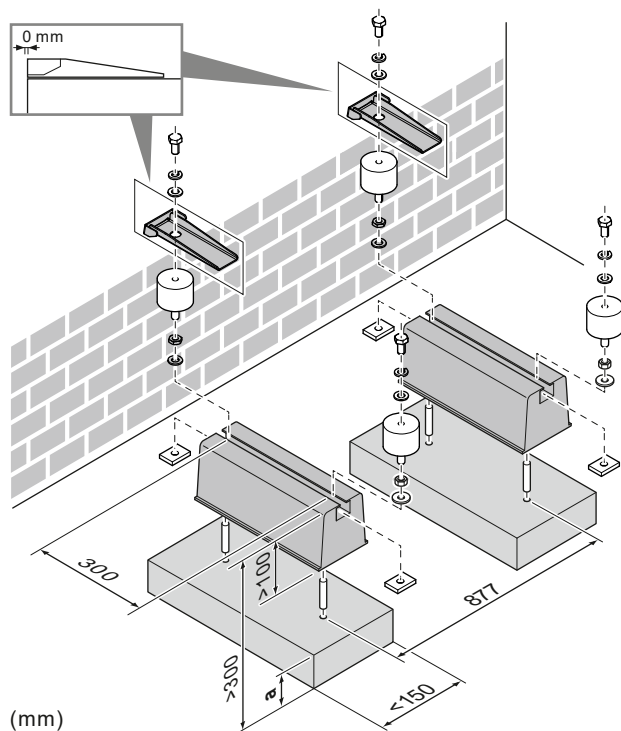
a Maksimālais sniega segas augstums
