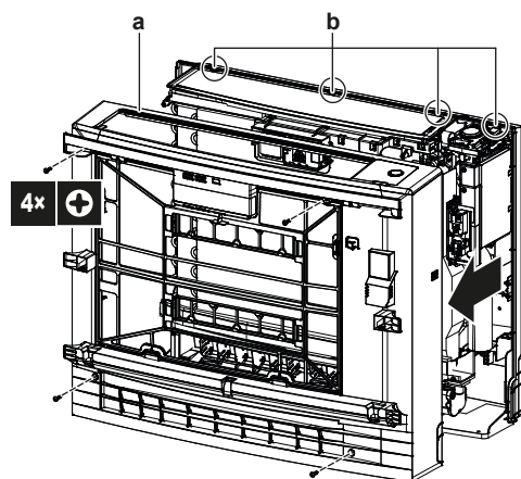
a Priekšējais režģis b Fiksatori
