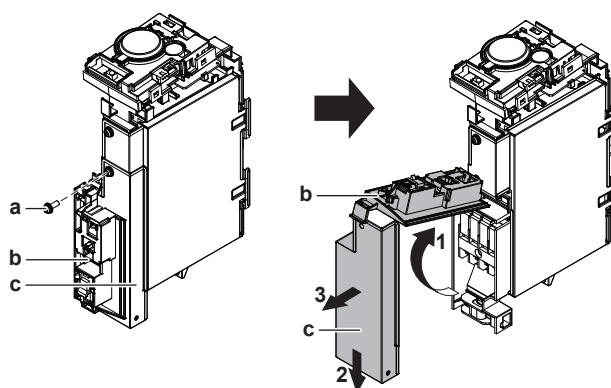
a Skrūve b Sensora piestiprināšanas plāksne c Metāla vāks
