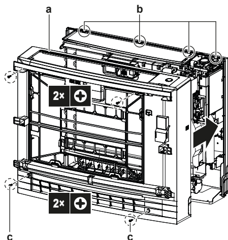
a Priekšējais režģis
