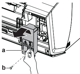
a Apkopes vāks b Apkopes vāka skrūve
