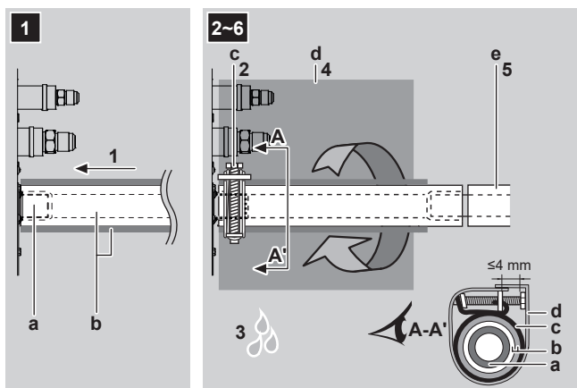
a Drenāžas cauruļvada savienojums (pie bloka) b Drenāžas šļūtene (piederums) c Metāla skava (piederums) d Lielais blīvējums (piederums) e Drenāžas cauruļvads (ārējais piederums)
